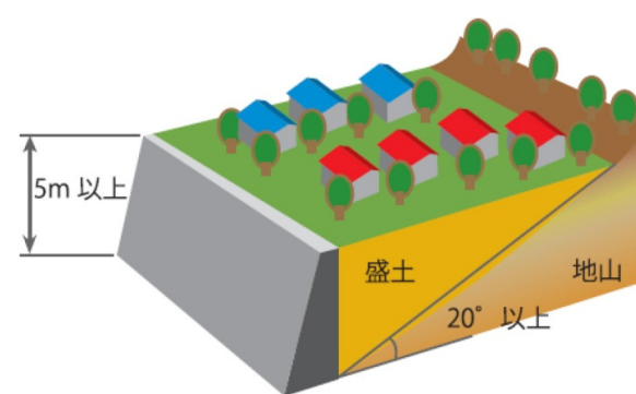
腹付け型
